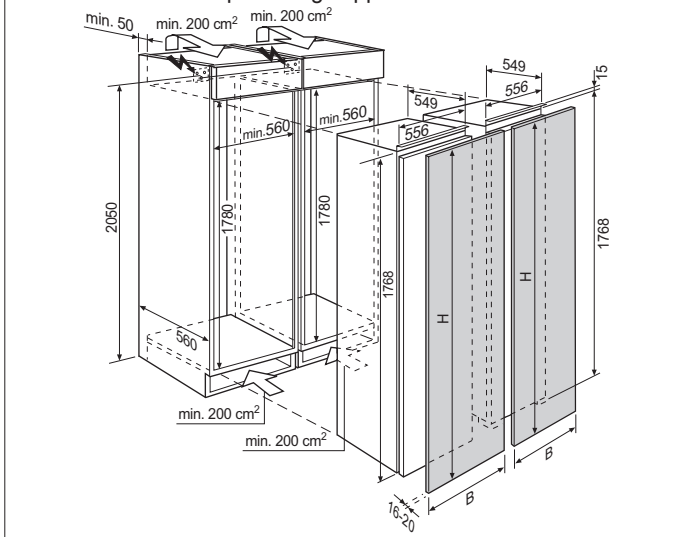
IK3035CZL e IG2085SN – incasso Euro Frontali avvitati sulle porte degli apparecchi
