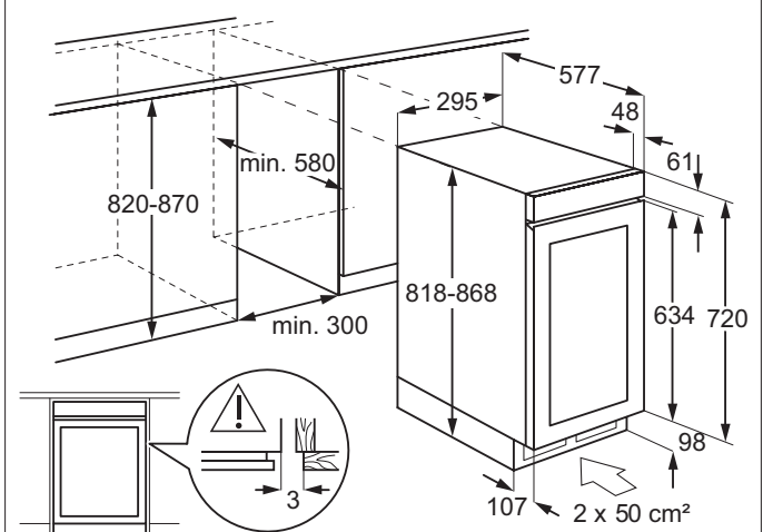
Armadio per vini sottobanco WKU30SSP
