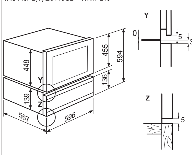
Cassetto scaldavivande/Cassetto accessori + Cantina per vini + Forno da incasso Compact da 45 VAC140PL(V)/ZS140GL + WK4PL10 + EB4... X
