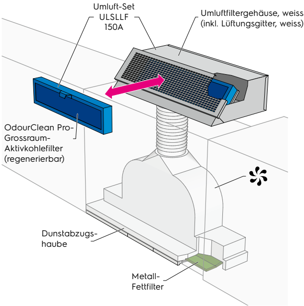
ULSLLF150A passend zu Oberschrank ohne Blende
