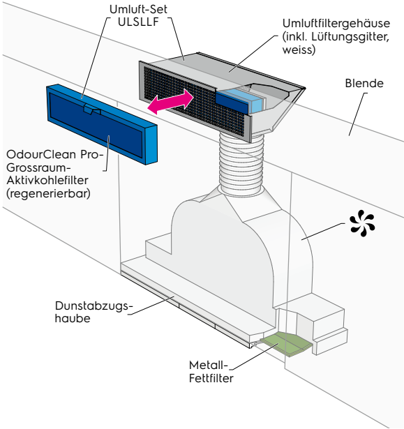
ULSLLF I ULSLLF125 passend zu Oberschrank mit Blende (Ausschnittmass 115 × 510 mm)
