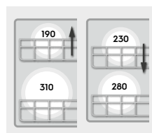
Maximale Tellergrößen EURO-Norm-Geschirrspüler mit 13 Massgedecken
