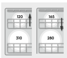
Maximale Tellergrößen EURO-Norm-Geschirrspüler mit 14/15 Massgedecken
