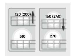
Maximale Tellergrößen 45 cm Geschirrspüler mit Besteckschublade und 10 Massgedecken (ohne Besteckschublade und 9 Massgedecken)
